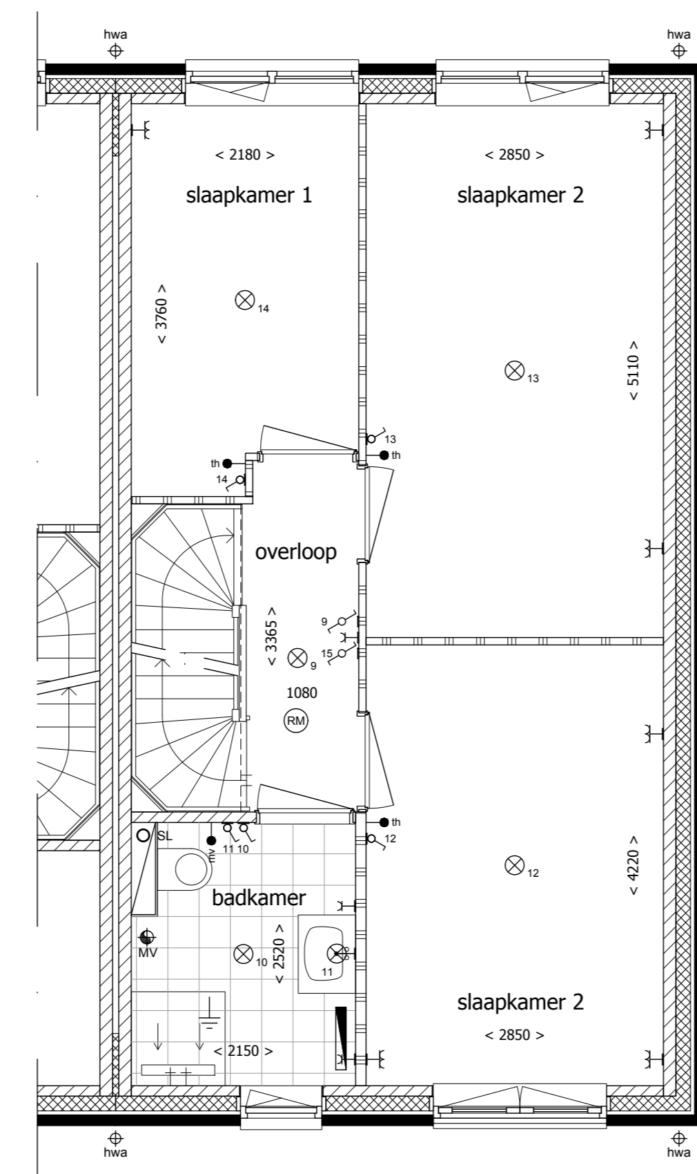
1e Verdieping
