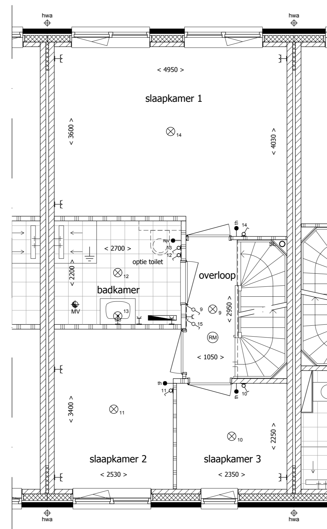
1e Verdieping
