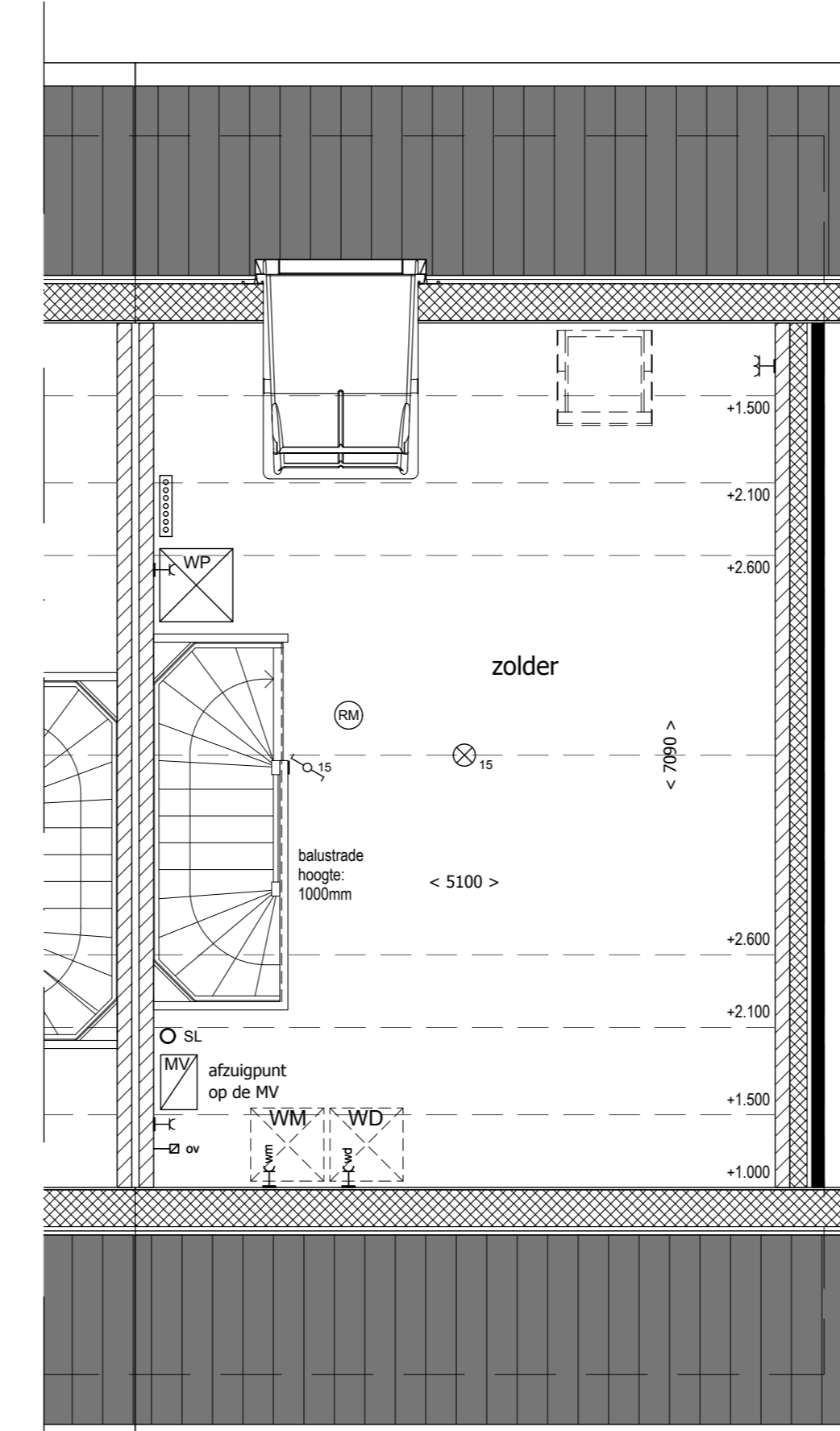
2e Verdieping
