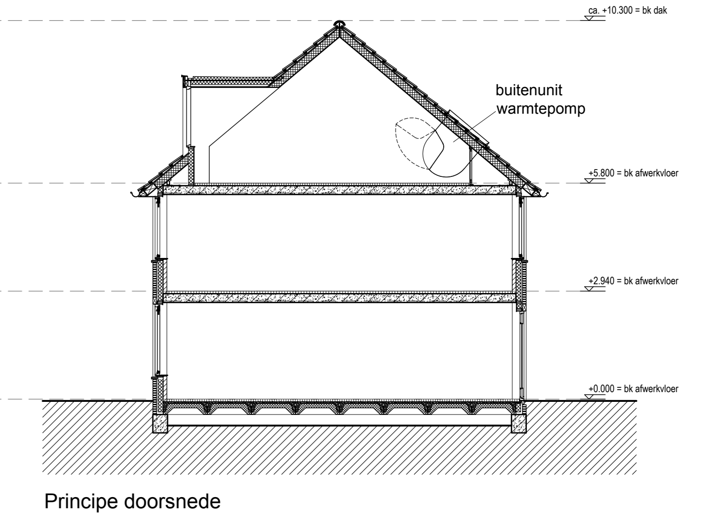
Principe doorsnede
