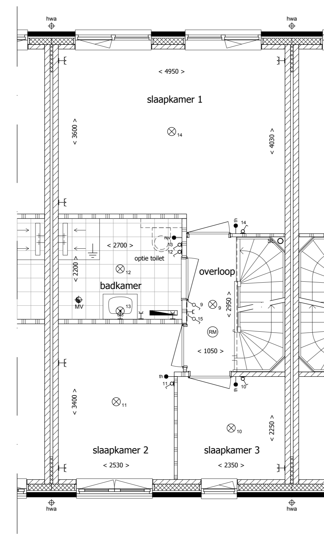
1e Verdieping
