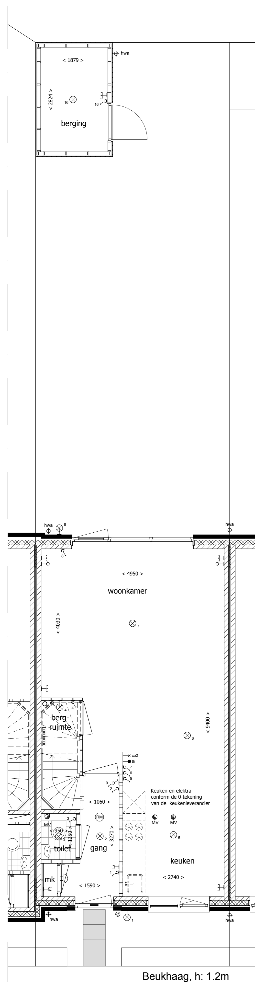
Begane grond
