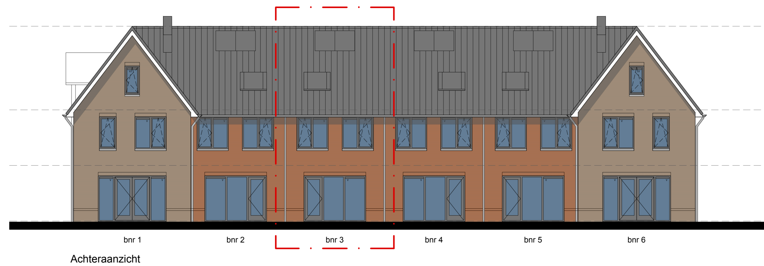
Achteraanzicht
