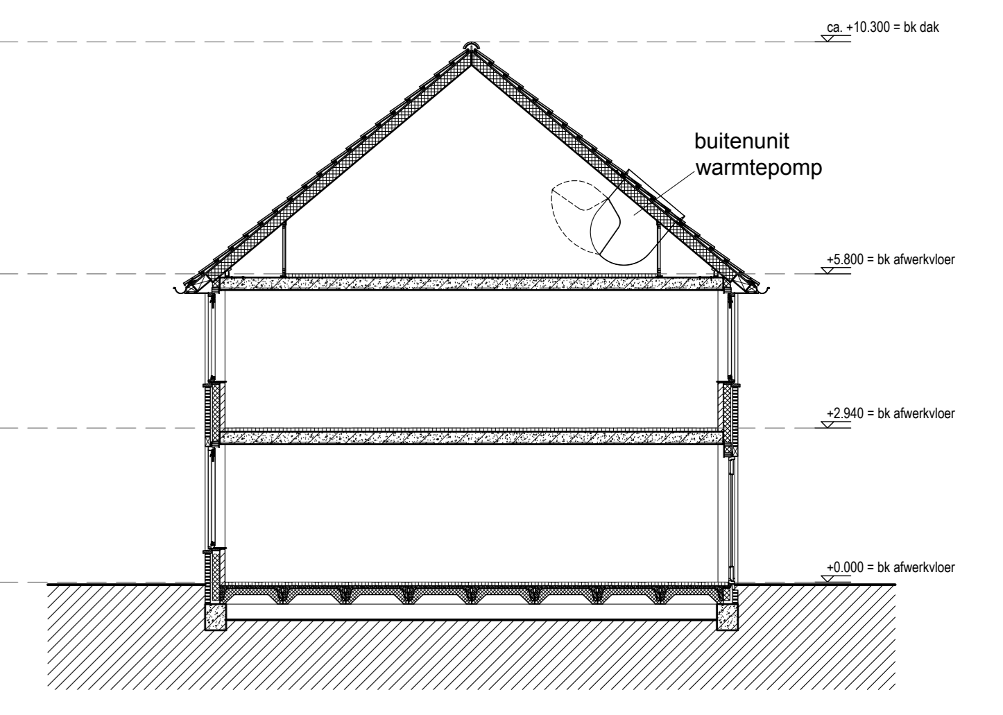
Principe doorsnede
