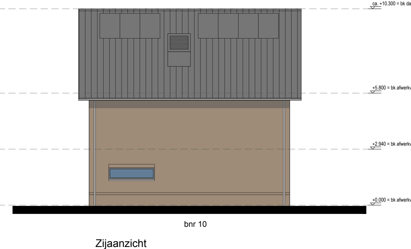
Zijaanzicht
